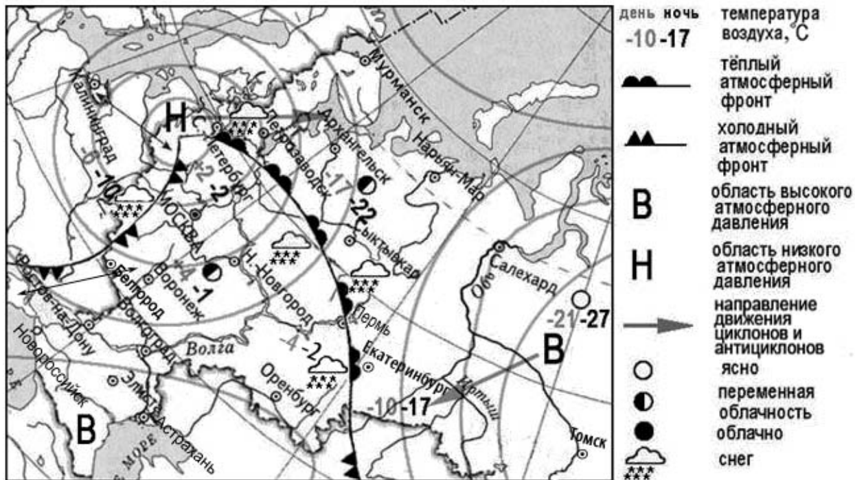
Карта прогноза погоды на 9 февраля (на 15 часов московского времени)
