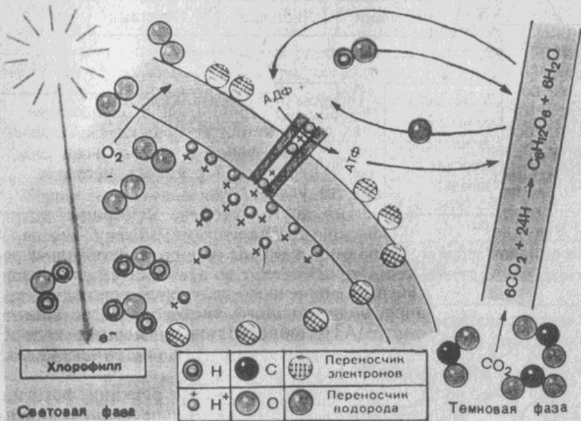
Схема фотосинтеза
